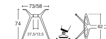
basamento con traversa mini base with mini cross bar
