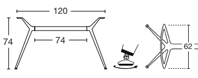
basamento con traversa lunga base with long cross bar
